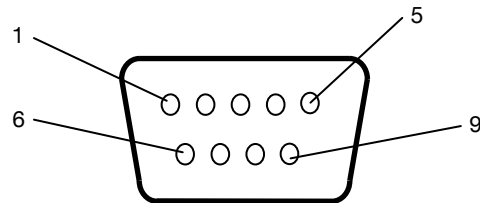
Mini D-SUB 9P
